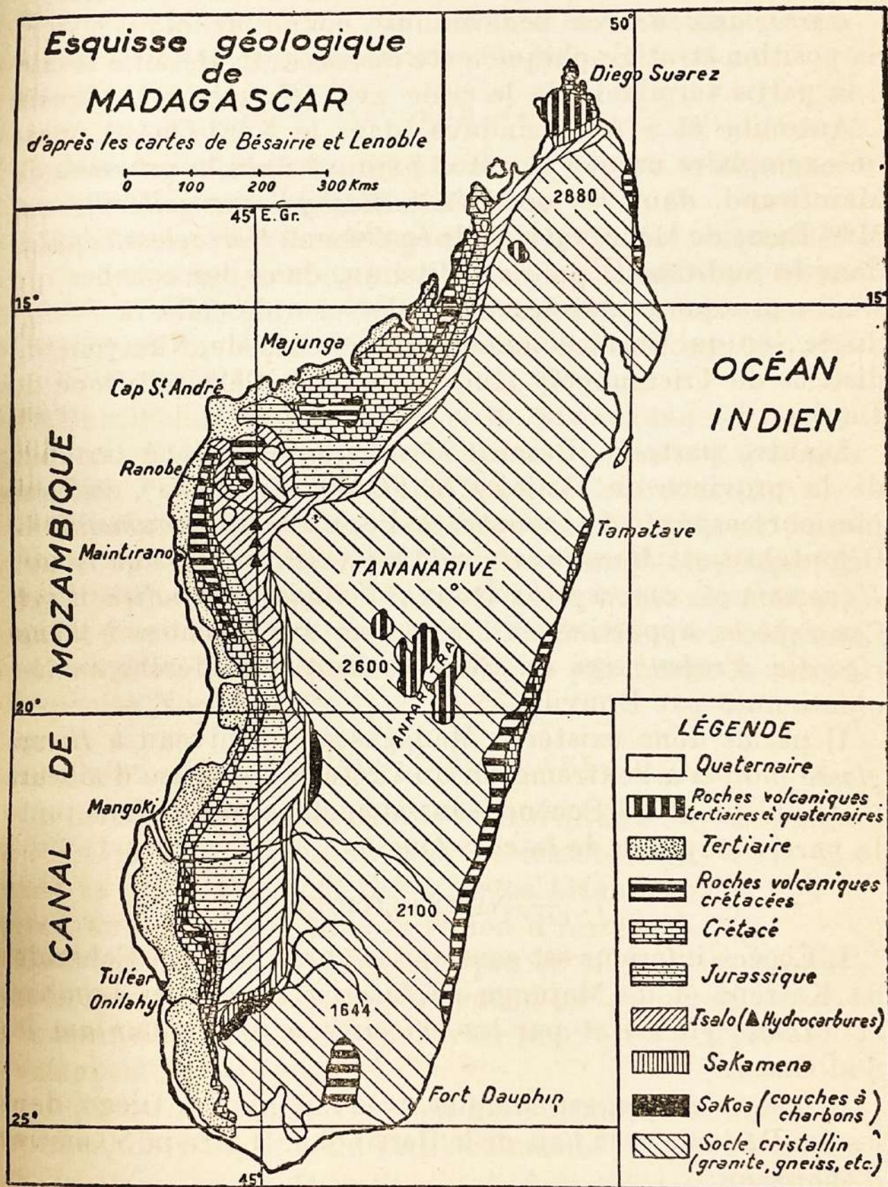
Fig. 34. — Croquis géologique de Madagascar (d'après H. Bésairie et A. Lenoble).
